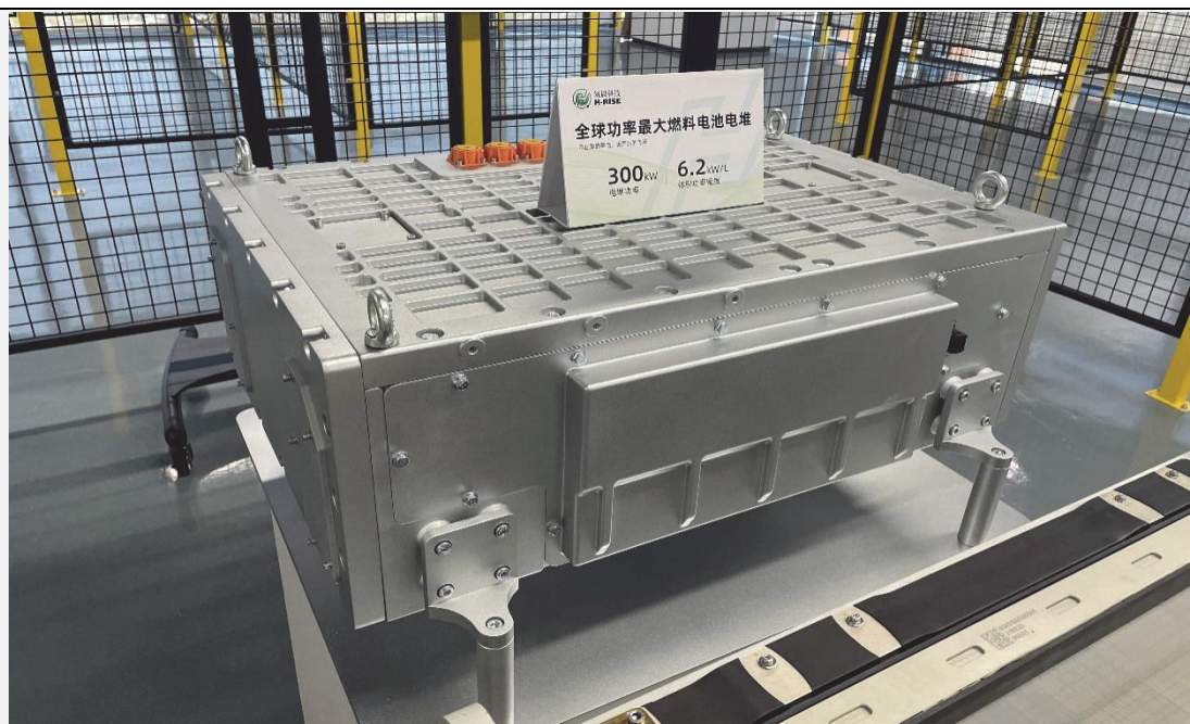
图 13 上海氢晨在 2022 年 8 月发布全球最大单堆 300 千瓦大功率燃料电池电堆
